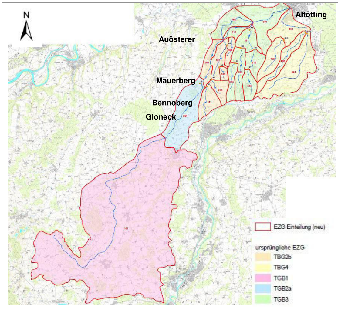
Abbildung 1: Einzugsgebiet Mörnbach (BCE-Modell 2012-2014)
